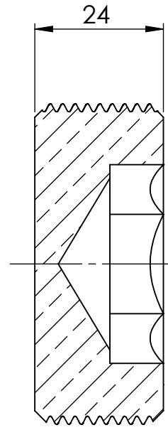
Ansicht / view A-A
