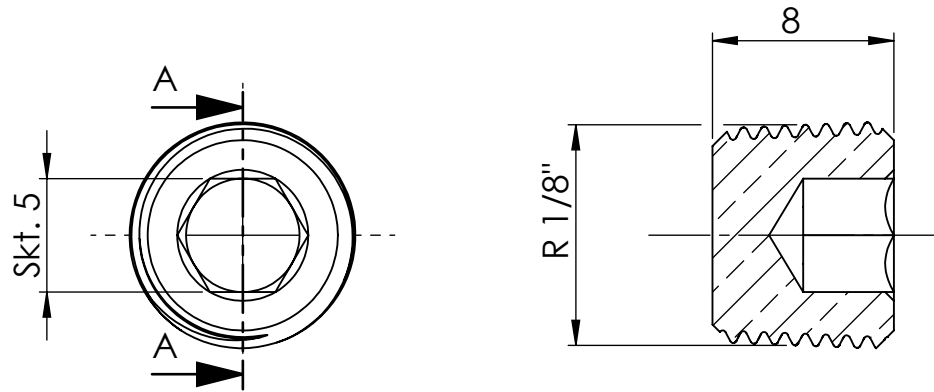
Ansicht / view A-A
