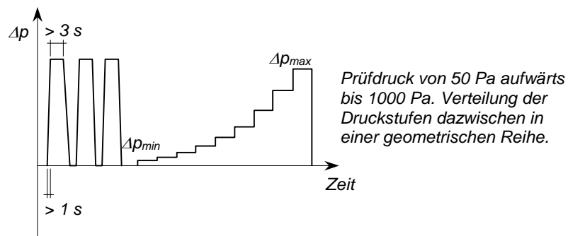
Abbildung 2 Prüfablauf (Druckfolge)
