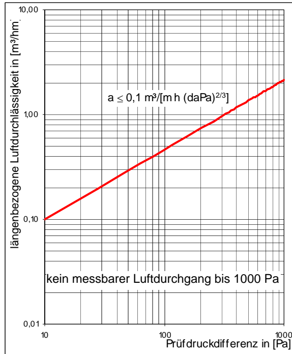
Diagramm 1 Längenbezogene Luftdurchlässigkeit des Montageschaums in einer „idealen“ Fuge mit einem Fugenquerschnitt von 20 mm x 60 mm
